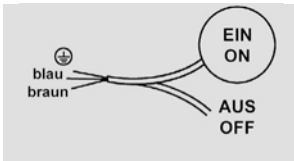
Schwimmschalter PSN-O zum Leerpumpen
