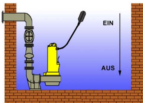
PSN-O Schwimmschalter zum Leerpumpen Schalter schließt in oberer Position und schaltet die Pumpe ein
