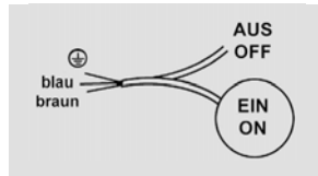
Schwimmschalter PSN-F zum Vollpumpen
