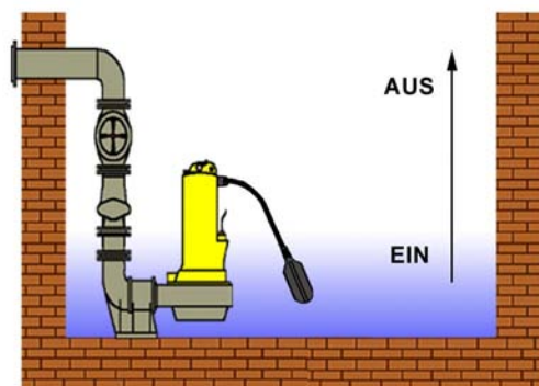
PSN-F Schwimmschalter zum Vollpumpen Schalter öffnet in oberer Position und schaltet die Pumpe aus
